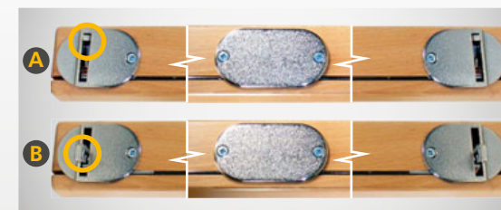
Dvojbodový zámok so zafrézovanými tiahkami
