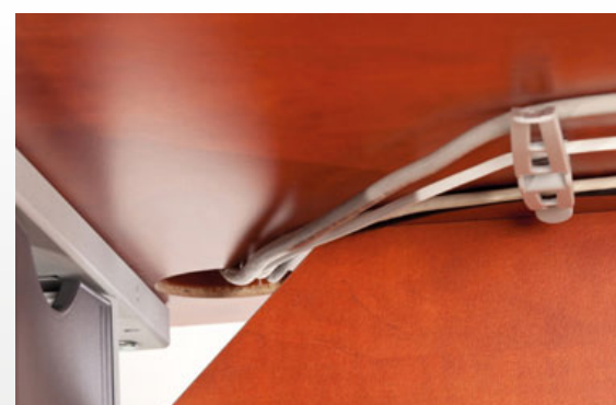
Káblové úchytky zabezpečujú praktické vedenie káblov pod pracovnou doskou
