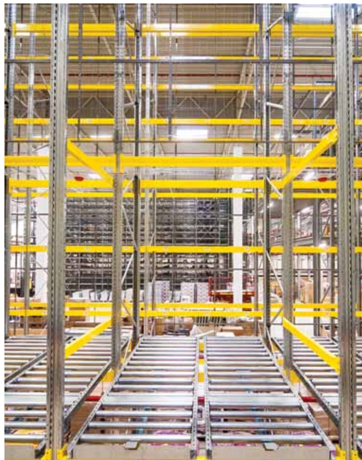
Spádové regály
