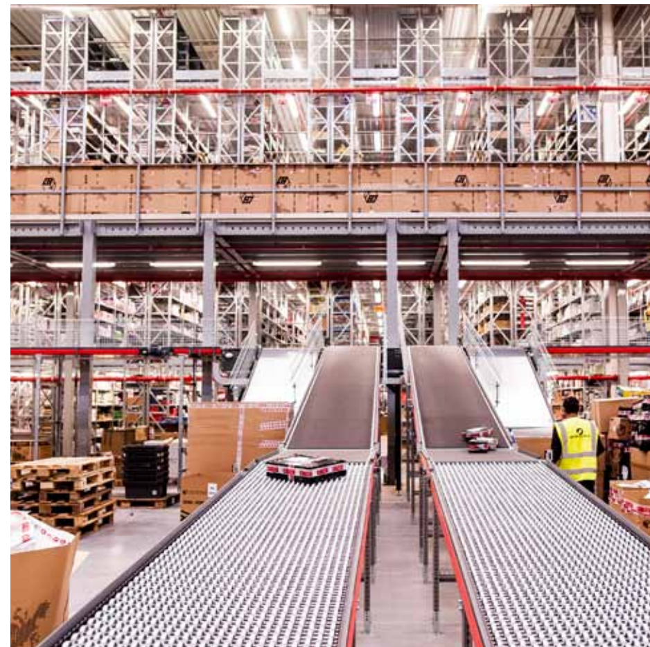
Válečkový dopravník
