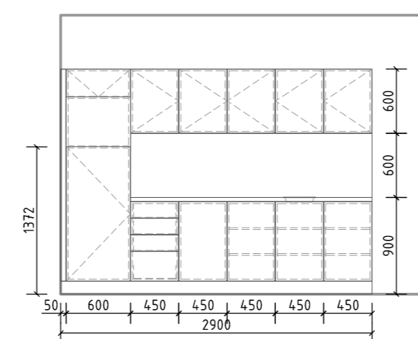
KUCH. LINKA miestnosť č. 1.17
